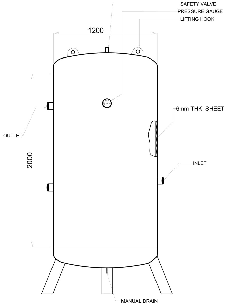
1 3000 Ltr AIR RECIEVER TANK Scale: NTS
