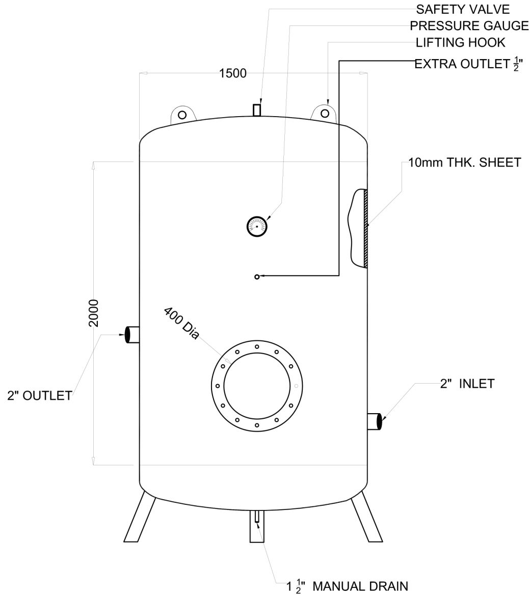
1 4000 Ltr AIR RECIEVER TANK Scale: NTS
