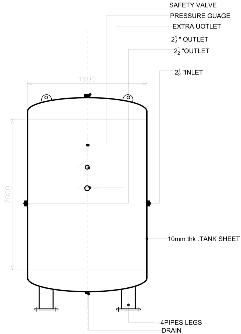
① 5000 Ltr AIR RECIEVER TANK Scale: NTS
